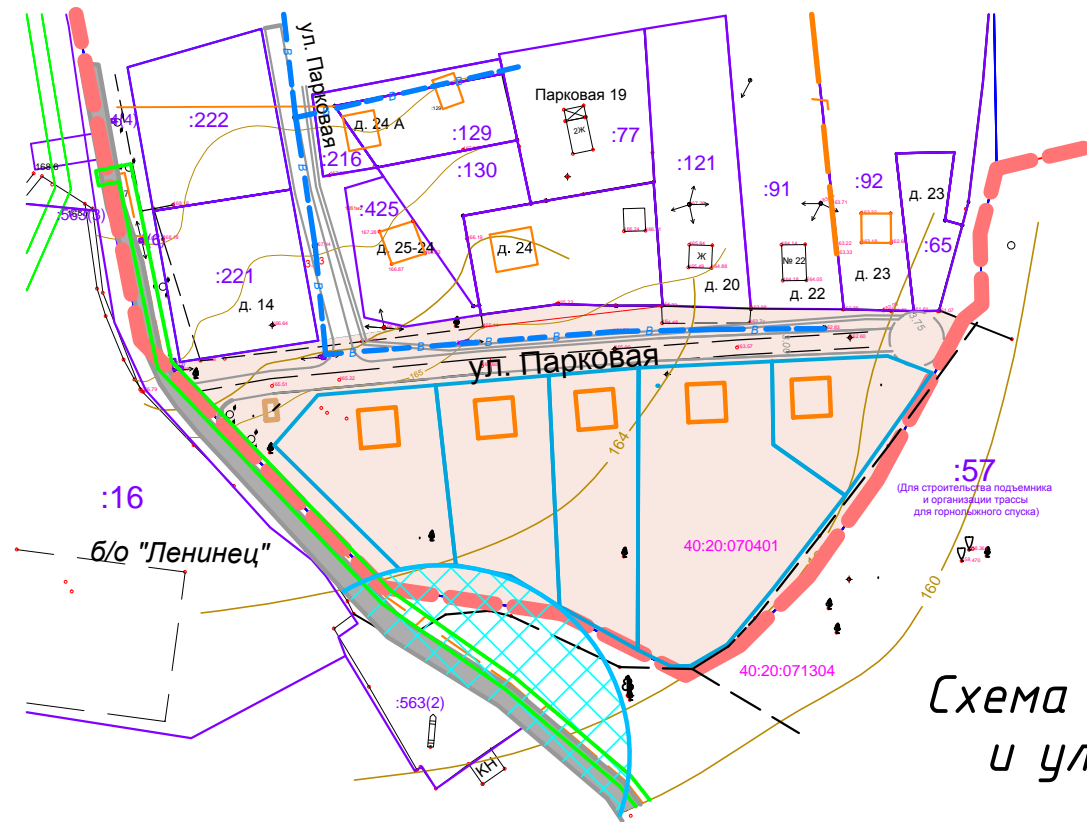
Схема размещения инженерных сетей Масштаб 1:2000
